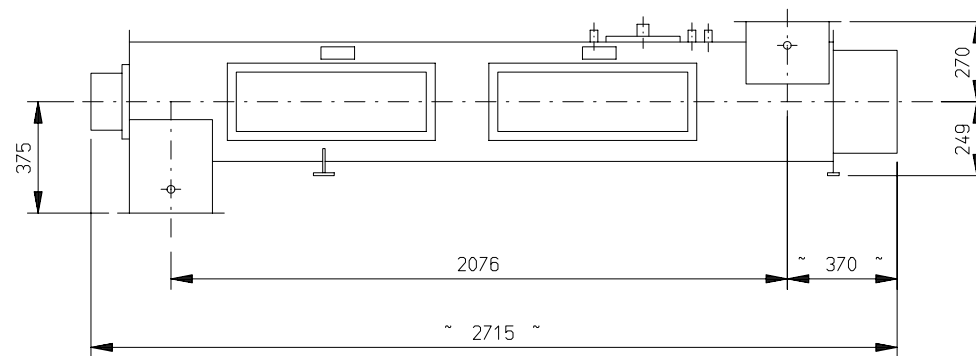
CONDITIONER 400X2400
